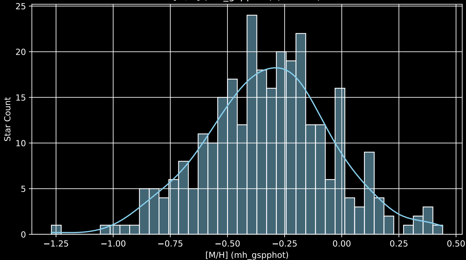
GALAH DR4 Field: [697] [M/H] (mh_gspphot) (n= 297)
