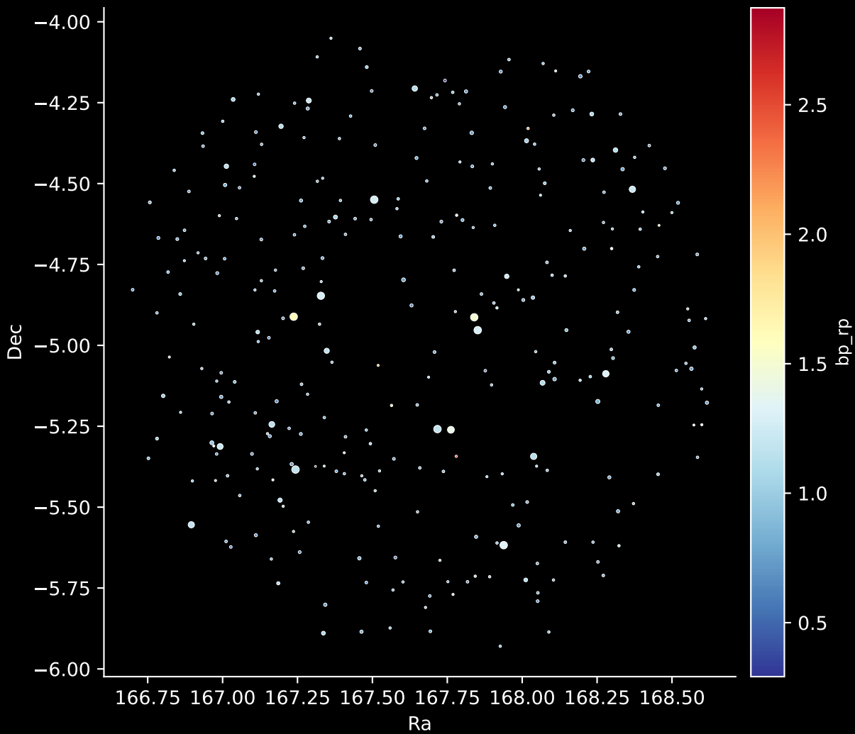
GALAH DR4 Field: [697] Stars: 297
