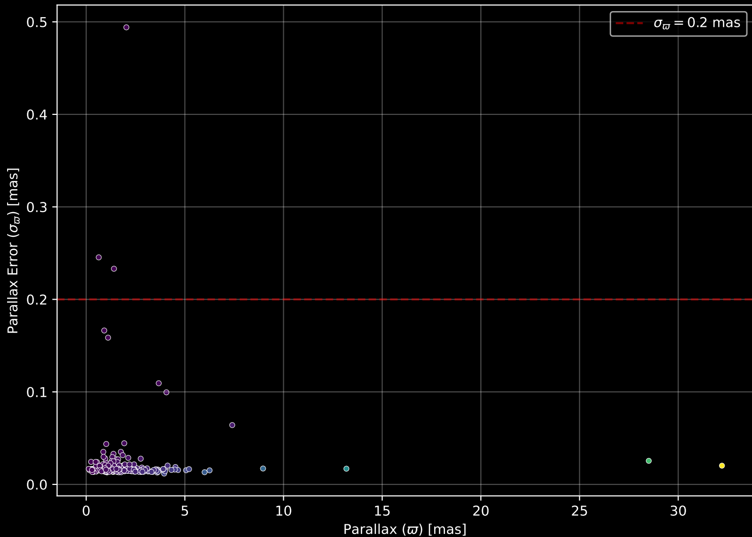
GALAH DR4 Field: [697] Parallax Quality (n= 297)
