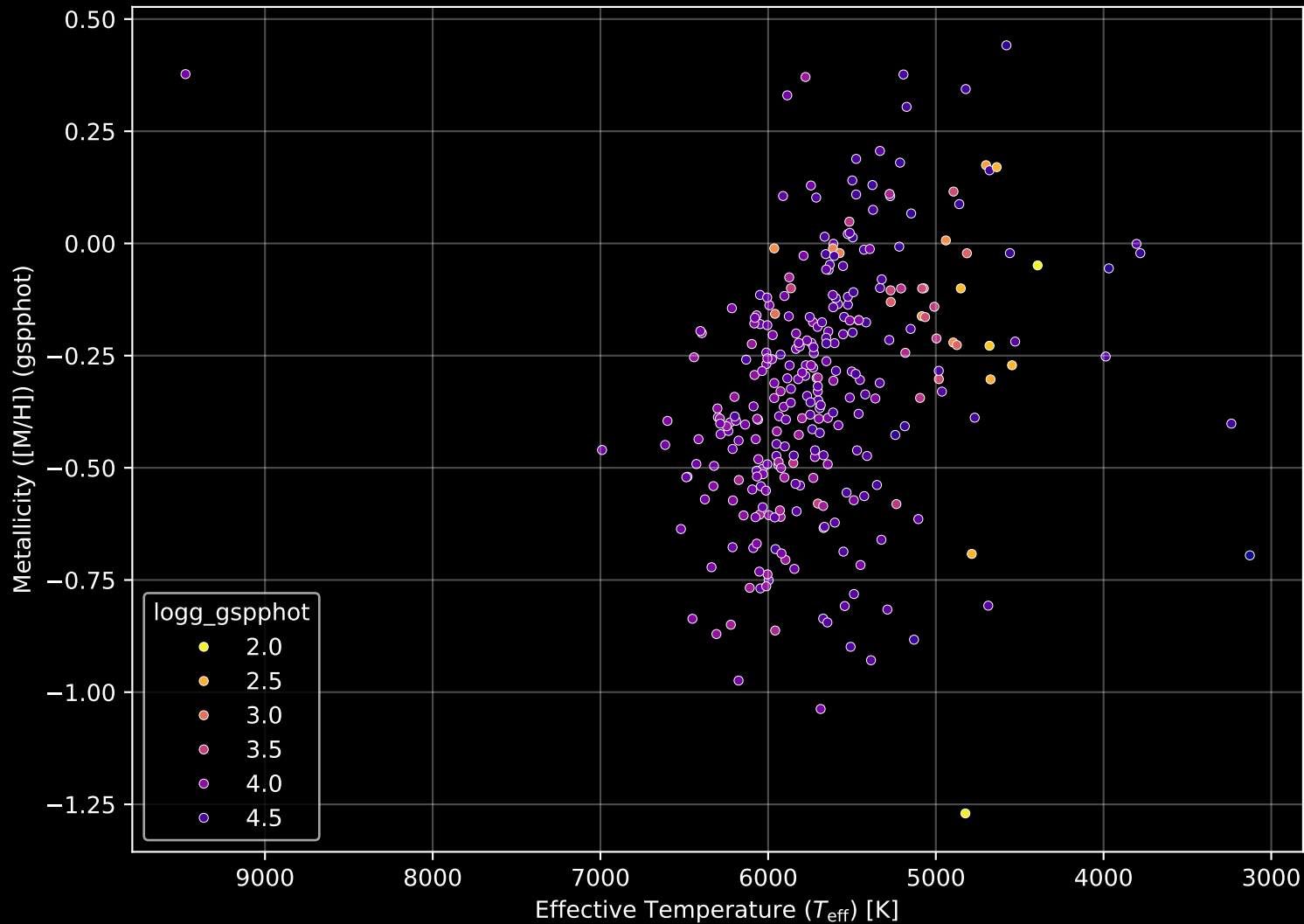
GALAH DR4 Field: [697] Stellar Population Parameters (n= 297)
